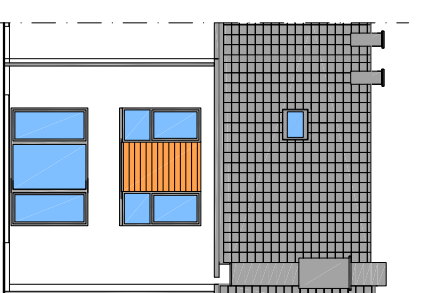
ELEWACJA POŁUDNIOWA
